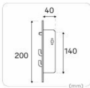
24005 Cerradura 9144 (T700)
